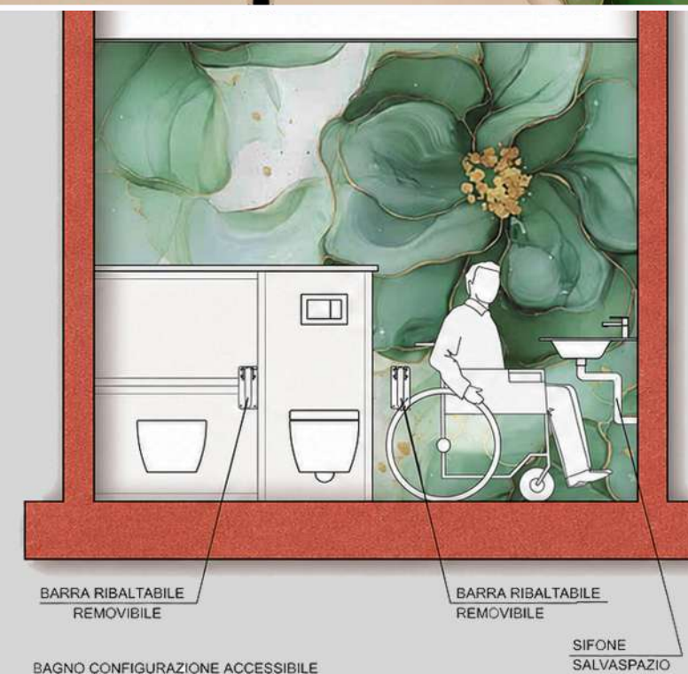
BAGNO CONFIGURAZIONE ACCESSIBILE
