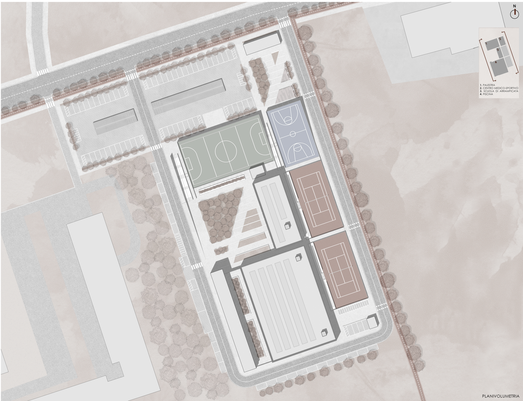
PLANIVOLUMETRIA
