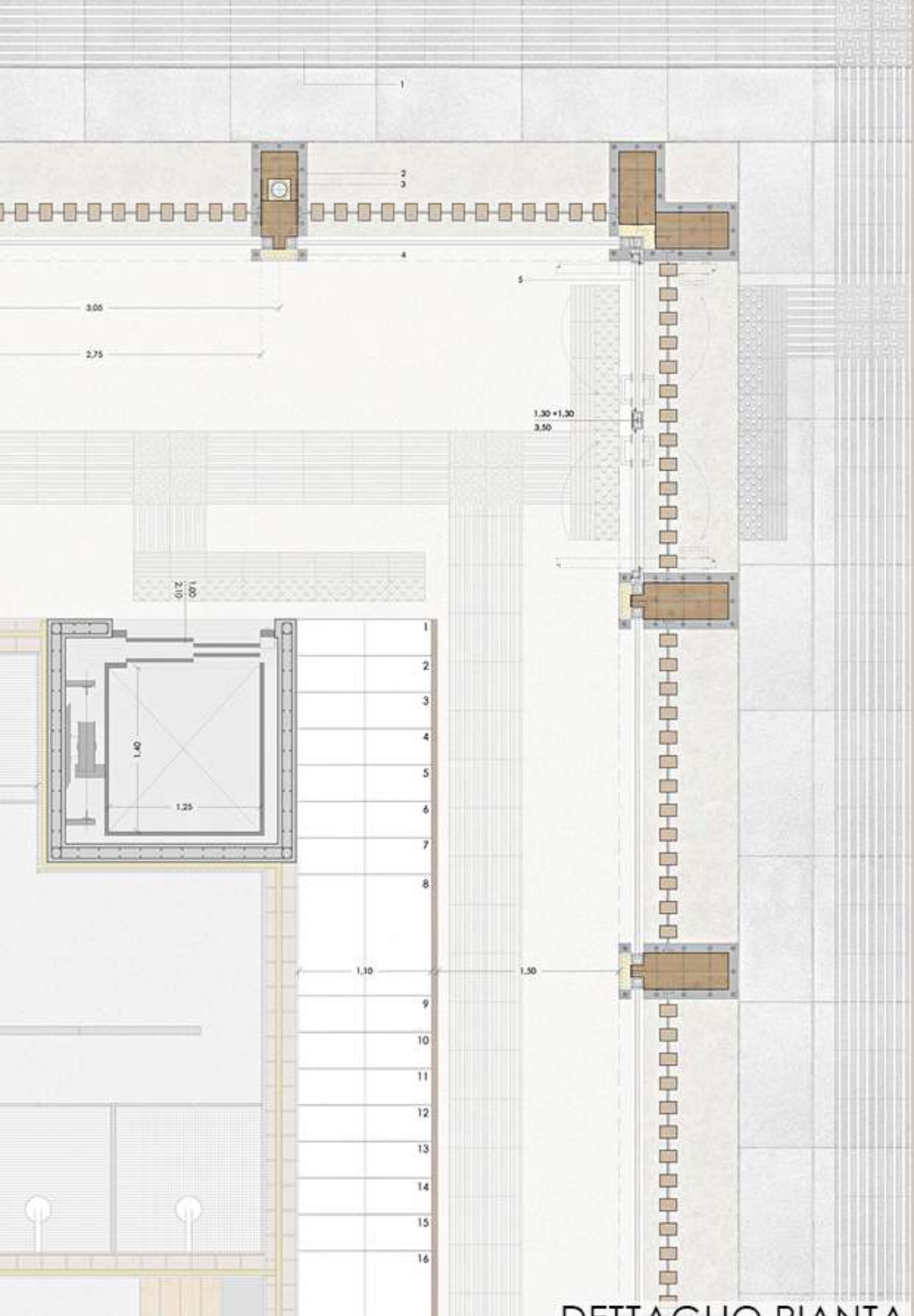
DETTAGLIO PIANTA
