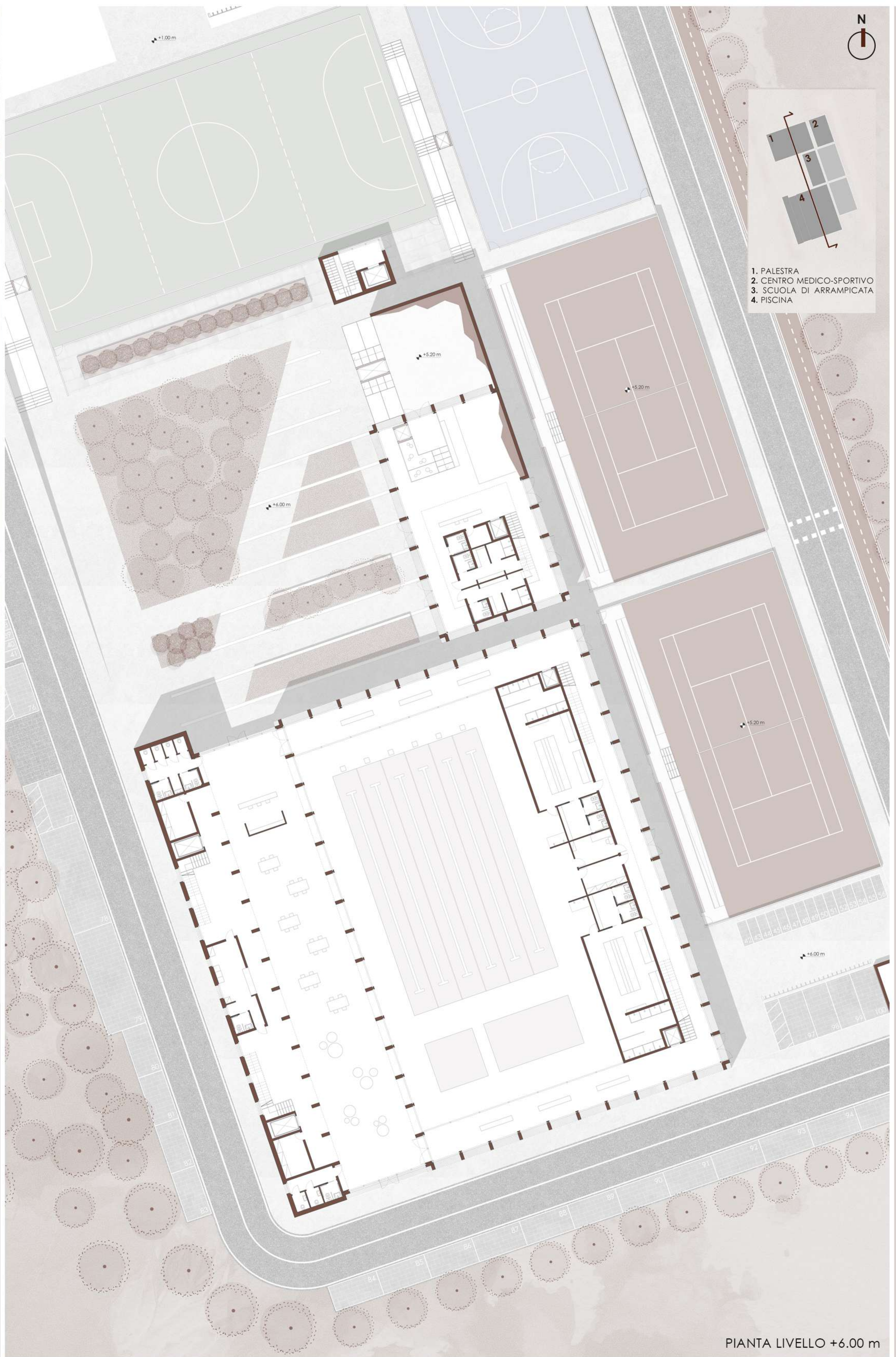
PIANTA LIVELLO +1.00 m
